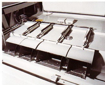
Dosing gates
